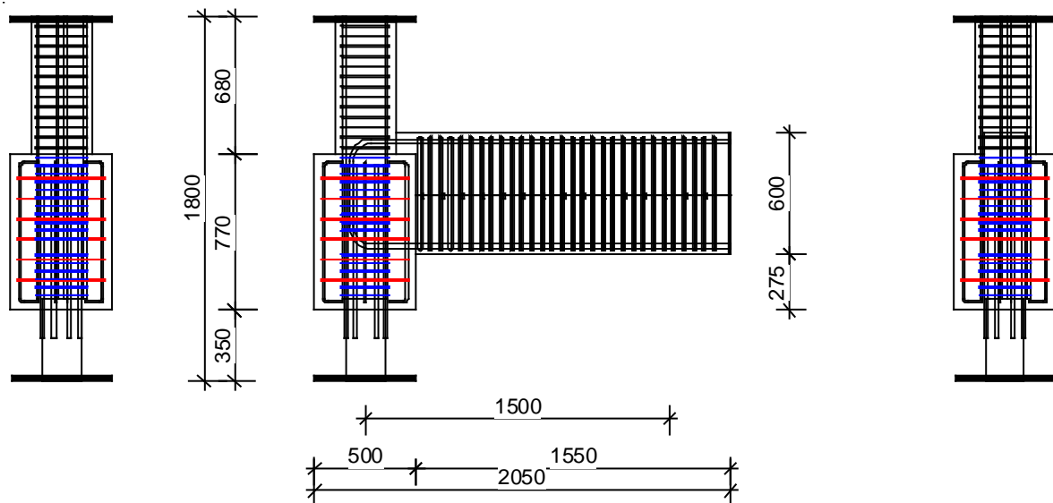
図2 試験体配筋図 (No,2 試験体)
