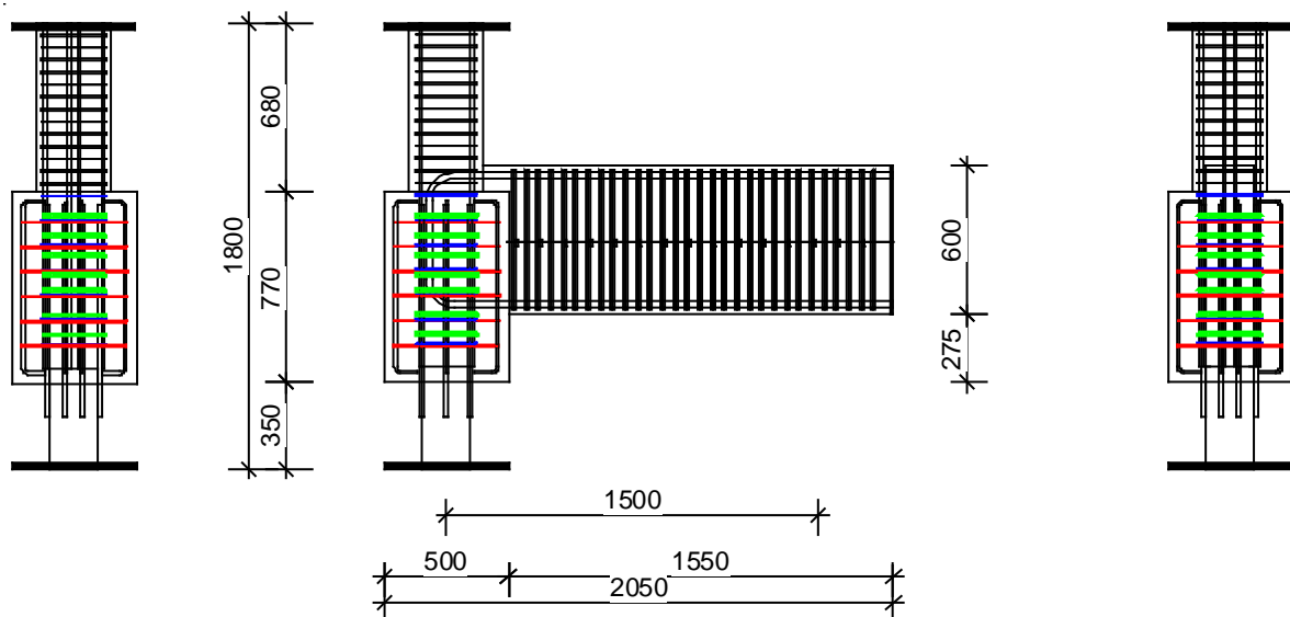
図3 試験体配筋図 (No,3 試験体)
