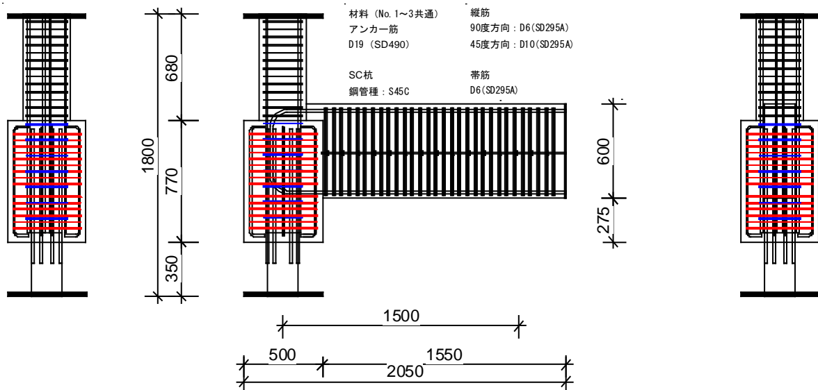
図1 試験体配筋図 (No,1 試験体)
