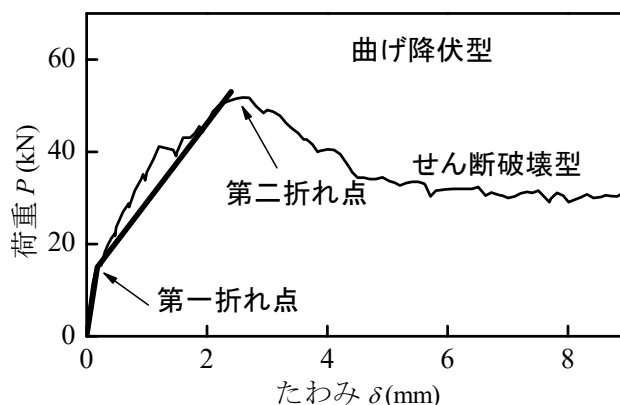
図 2.3.4 せん断破壊型の荷重－変形関係とそのモデル化
