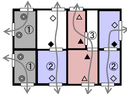
図1 通風経路①～③
