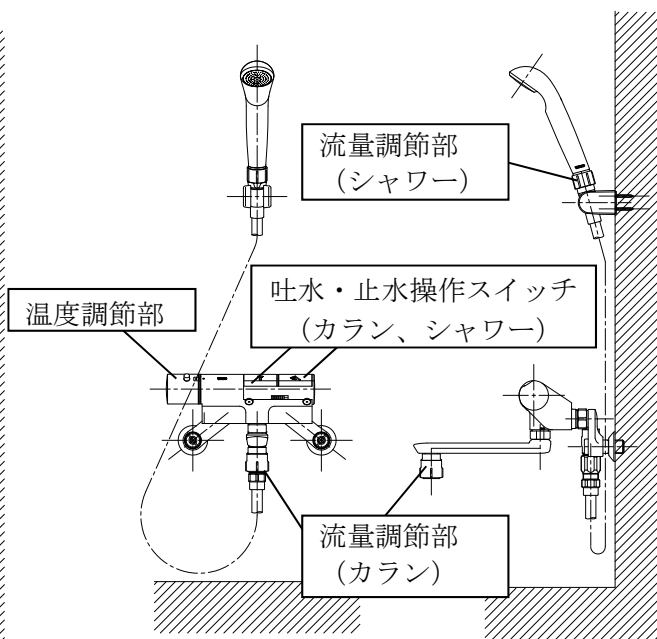
図 2-4.6手元止水機能の例2
