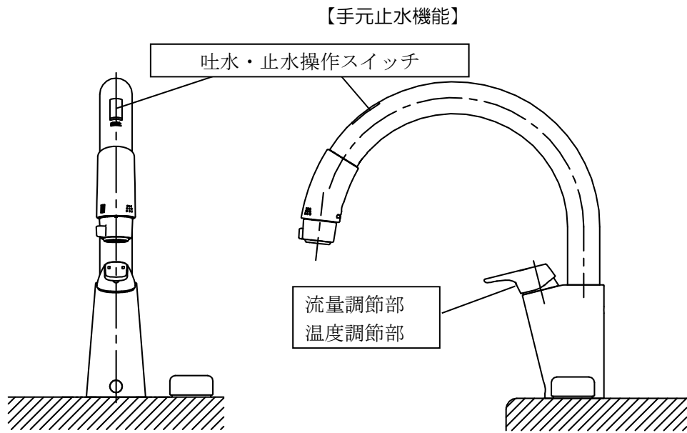
図 2-4.1 手元止水機能の例1
