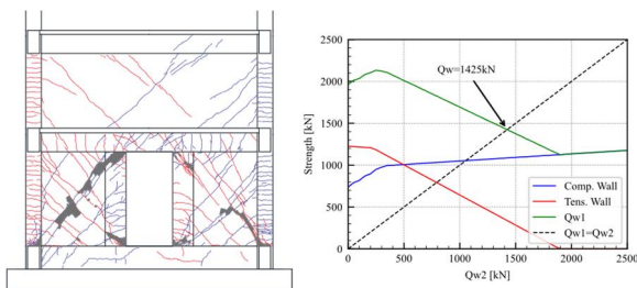
図2 実大2.5層RC耐力壁架構の構造実験と耐力評価
