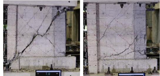
図3 新設開口横の片側柱付きRC耐力壁の構造実験
