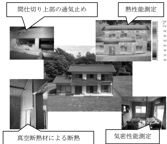
図 4 建築ストックへの適用に関する実験
