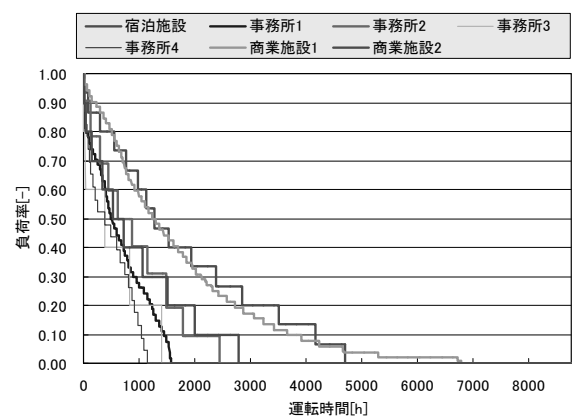
図 5 事務所等における部分負荷発生状況(冷熱)の例
