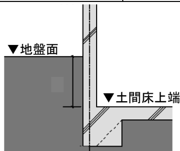
図 2 土間床上端が地盤面より低い場合の土間床上端と地盤面の高さの差
